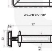
З'ЄДНУВАЧ 90°
