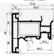
ШТУЛЬП
