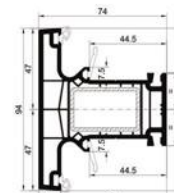
ІМПОСТ 94мм
