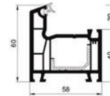
РАМА 60мм
