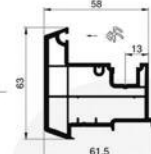
ФАЛЬШІМПОСТ (ШТУЛЬП)
