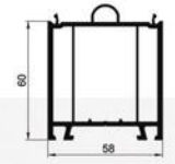
РОЗШИРЮВАЧ 60
