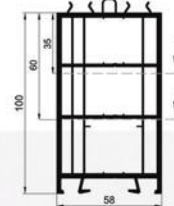
РОЗШИРЮВАЧ 100
