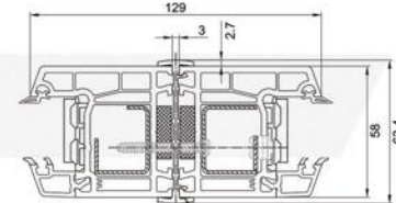
ІМПОСТ 80мм
