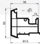
ШТУЛЬПА
