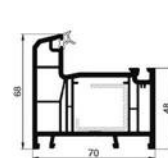
РАМА 68мм
