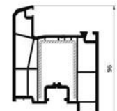
СТУЛКА ДВЕРНА Z 96мм
