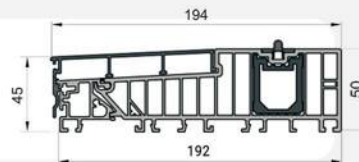
ПОРІГ
