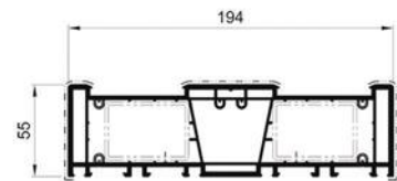
РАМА
